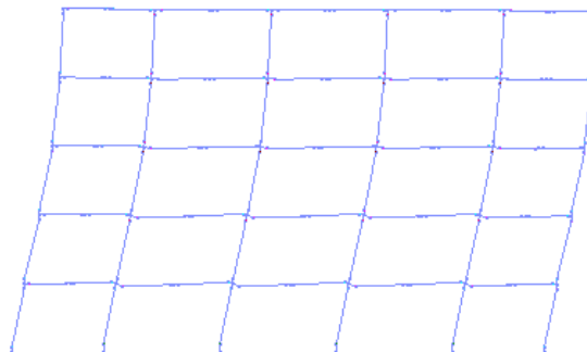
Figura 7. Simulación del análisis Pushover en OpenSees [18].
