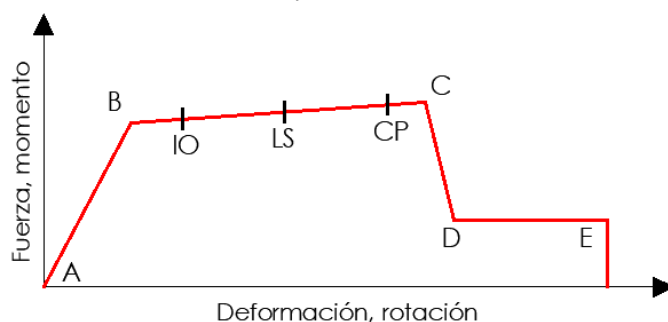
Figura 11. Gráfica fuerza vs deformación [19].
