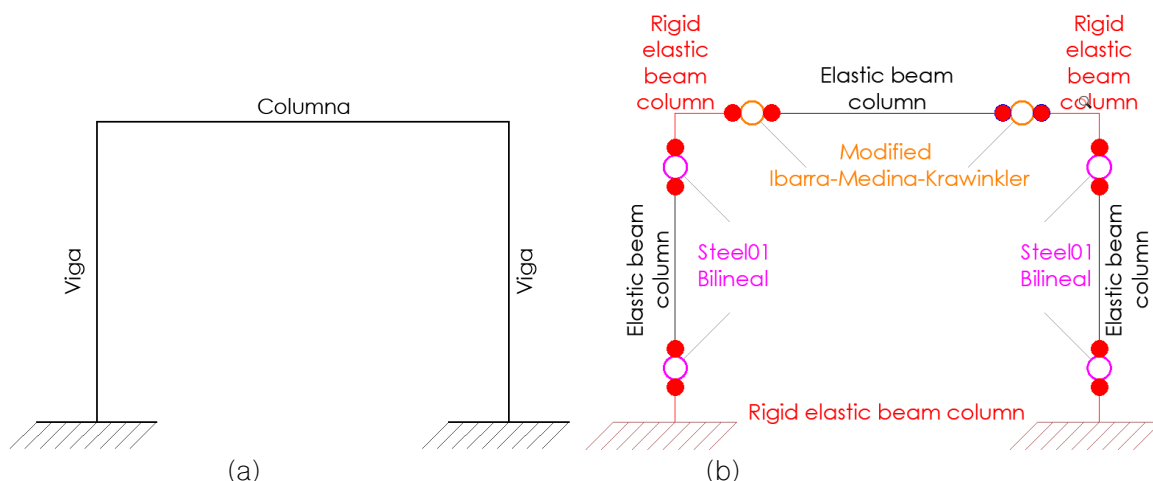
Figura 4. a) Modelo generado en CEINCI-LAB; b) Modelo con zonas de plasticidad concentrada y elementos elásticos para el análisis Pushover no lineal en OpenSees [6].
