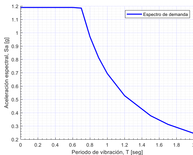
Figura 22. Espectro de demanda
