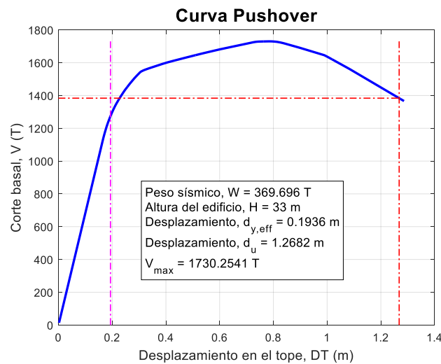
Figura 20. Curva de capacidad del pórtico SMF de 10 niveles, en el eje "x".
