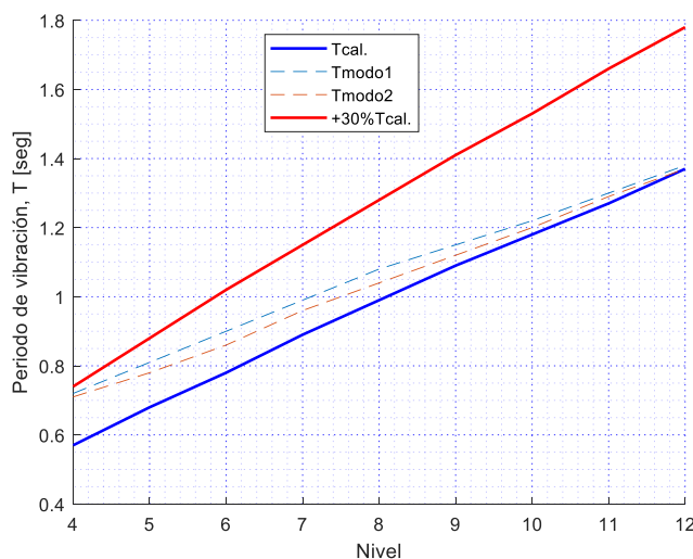
Figura 13. Periodo de vibración vs Número de niveles, edificaciones 3D.
