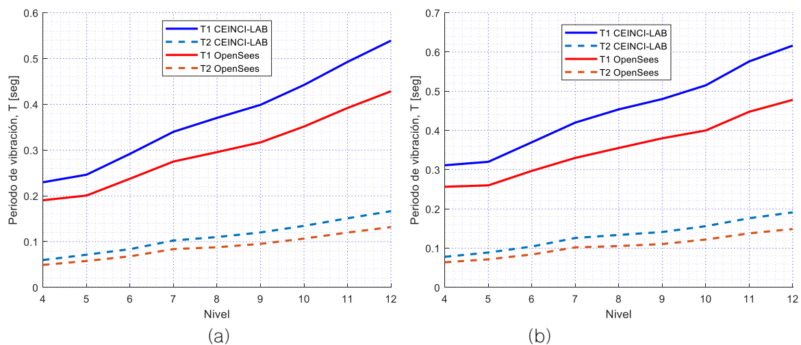
Figura 19. Periodo de vibración vs. Número de niveles, a) eje "x", b) eje "y". Pórticos SMF (2D).
