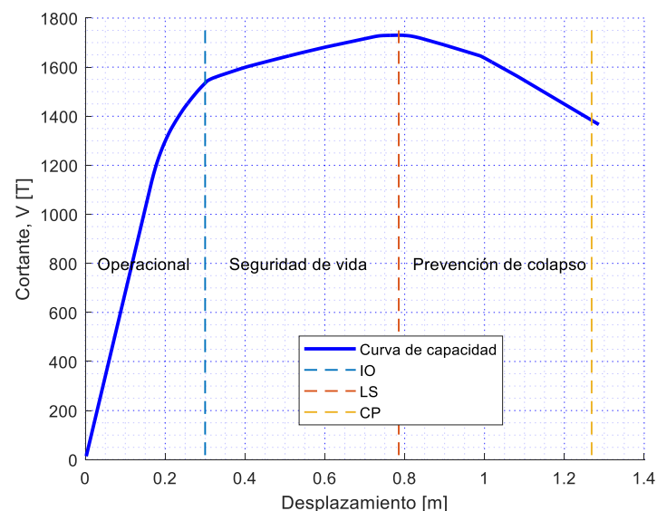
Figura 24. Curva de capacidad con niveles de desempeño. Pórtico de 10 niveles, eje “y”.
