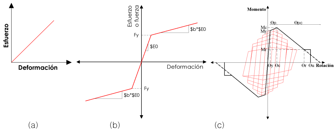
Figura 5. Constitutivas; a) modelo de elemento elástico; b) Steel01 Material , comportamiento histerético del modelo elastoplástico, para articulaciones en columnas; c) modelo modificado de deterioro de Ibarra Medina y Krawinkler (IMK) , para articulaciones en vigas [7].
