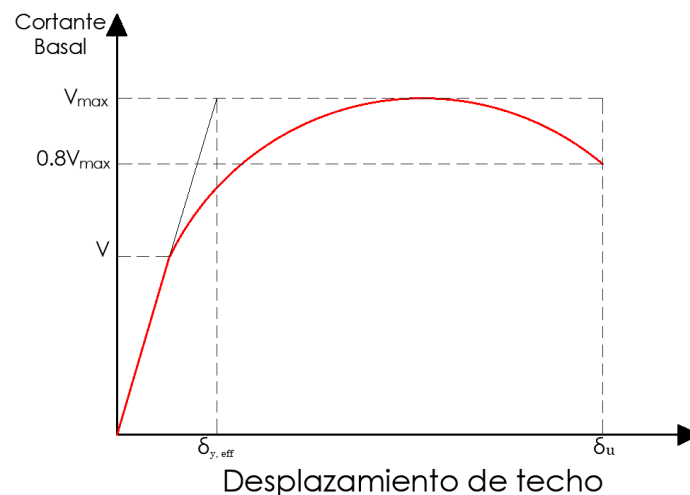
Figura 9. Curva Pushover idealizada [19].
