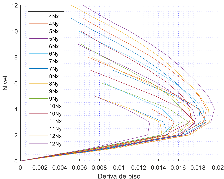
Figura 14. Número de niveles vs. Deriva de piso en el eje "x" e "y", edificaciones 3D.
