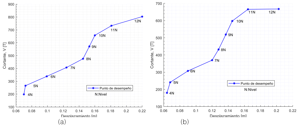
Figura 23. Puntos de desempeño: a) pórticos eje “x”, b) pórticos eje “y”
