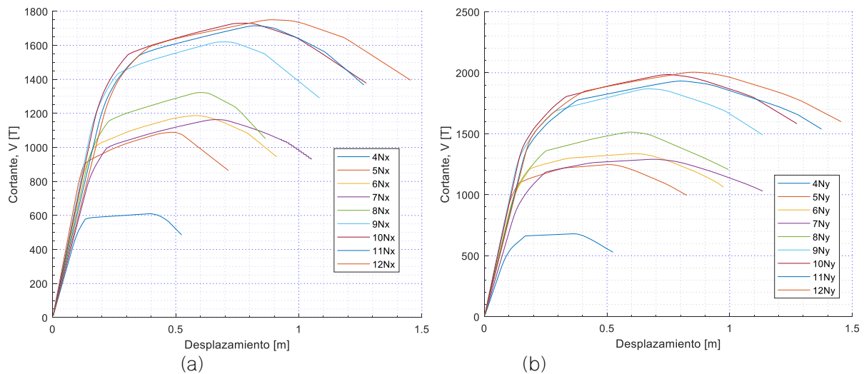
Figura 21. Curva de capacidad, a) pórticos eje "x", b) pórticos eje "y".
