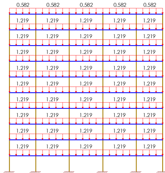
Figura 15. Pórtico SMF de 10 niveles cargado, eje "x" [T/m].
