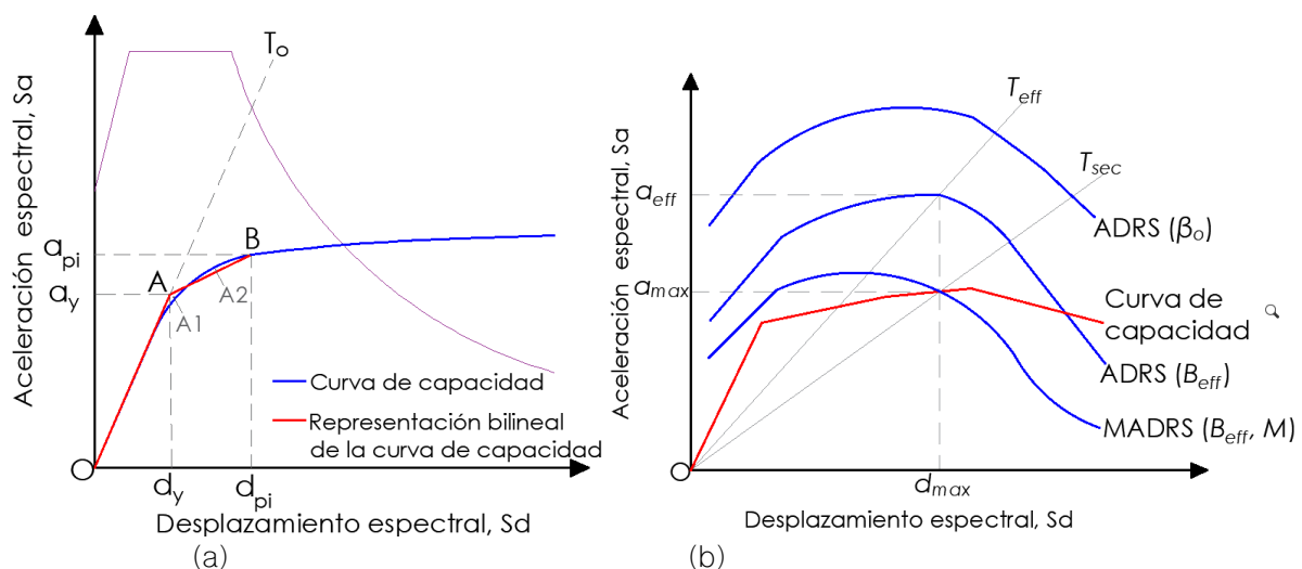
Figura 10. a) Representación bilineal de la curva de capacidad; b) Espectro modificado de respuesta (MADRS) para obtener el punto de desempeño con el periodo secante, T_{sec} [23].
