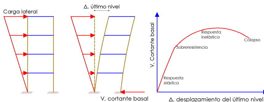
Figura 3. Secuencia de análisis Pushover [3].
