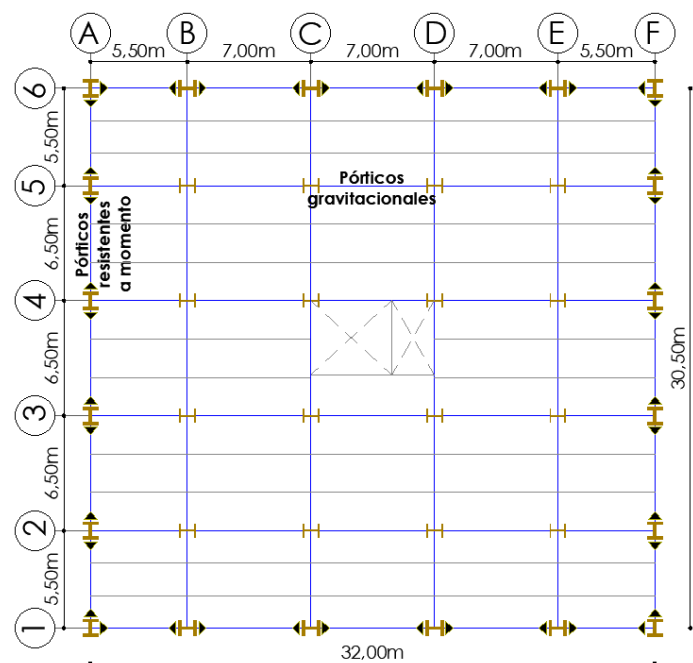
Figura 12. Planta, modelo de edificación.
