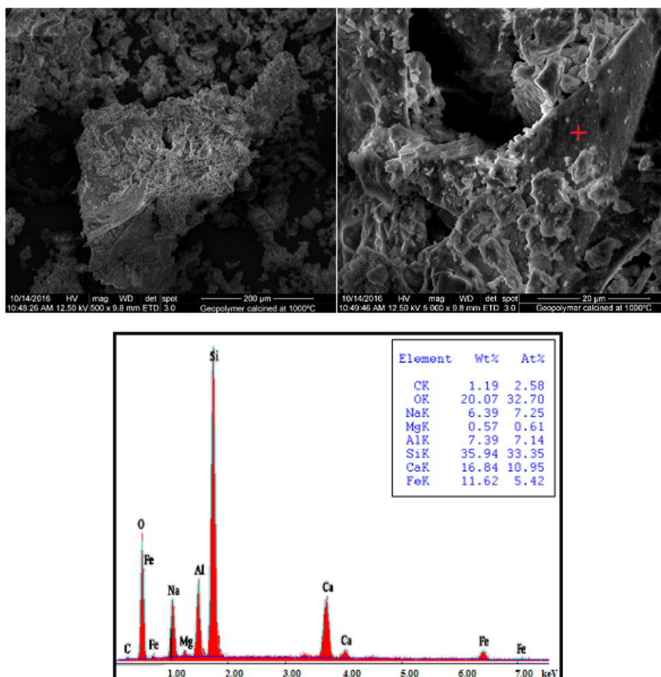
Figura 4. Micrografías SEM del geopolímero calcinado a 20°C/min
